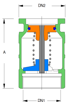
Tappo 1610
